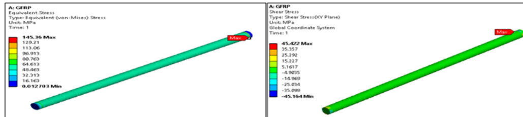
Fig.7-Equivalent Stresses
