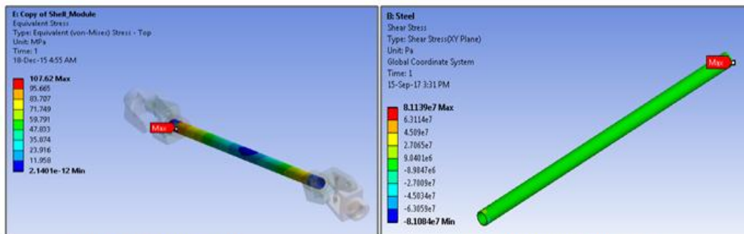
Fig.3-Equivalent Stresses
