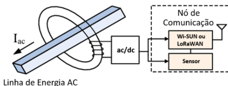
Figura 5 - Coleta de Energia por Campo Eletromagnético (topologia de núcleo fixo).
